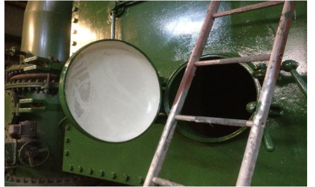
Kondanse iç yüzeyleri EURO COAT 1348 T ile kaplanmış hali
