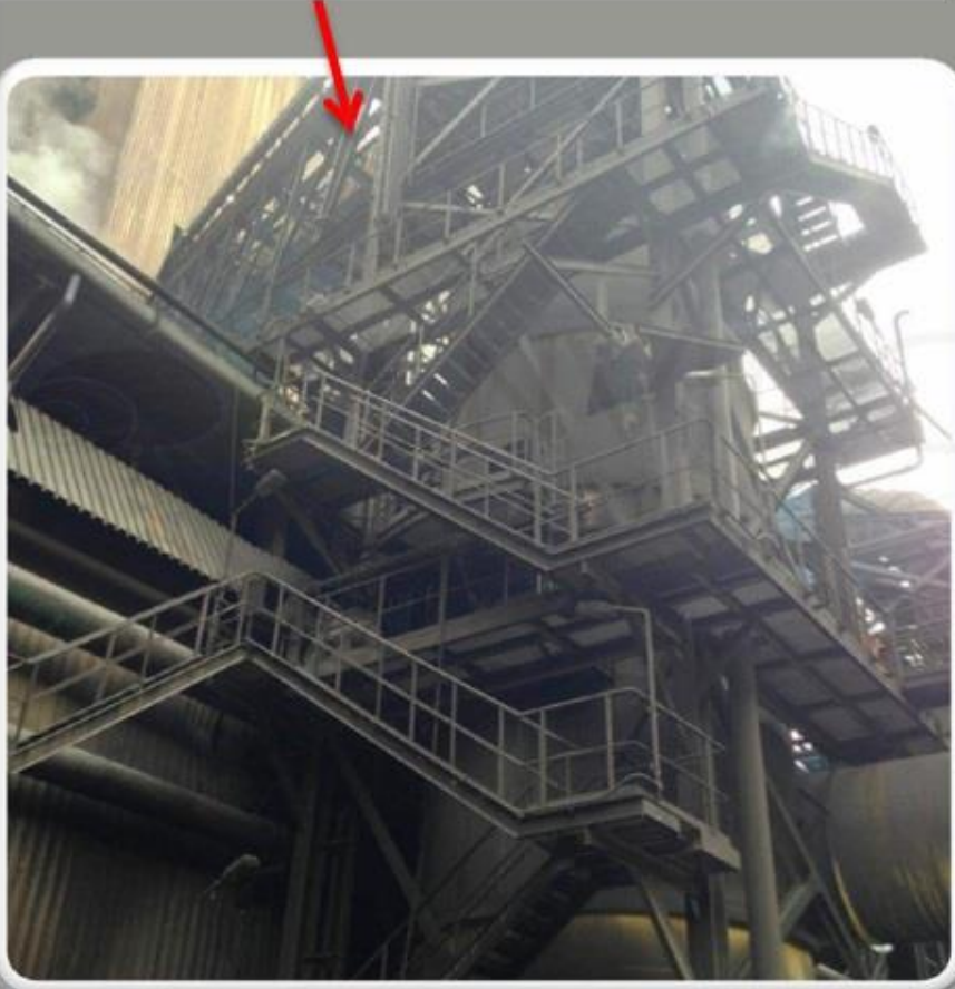
İsdemir Dikey Baca Sucrubber Ünitesi
