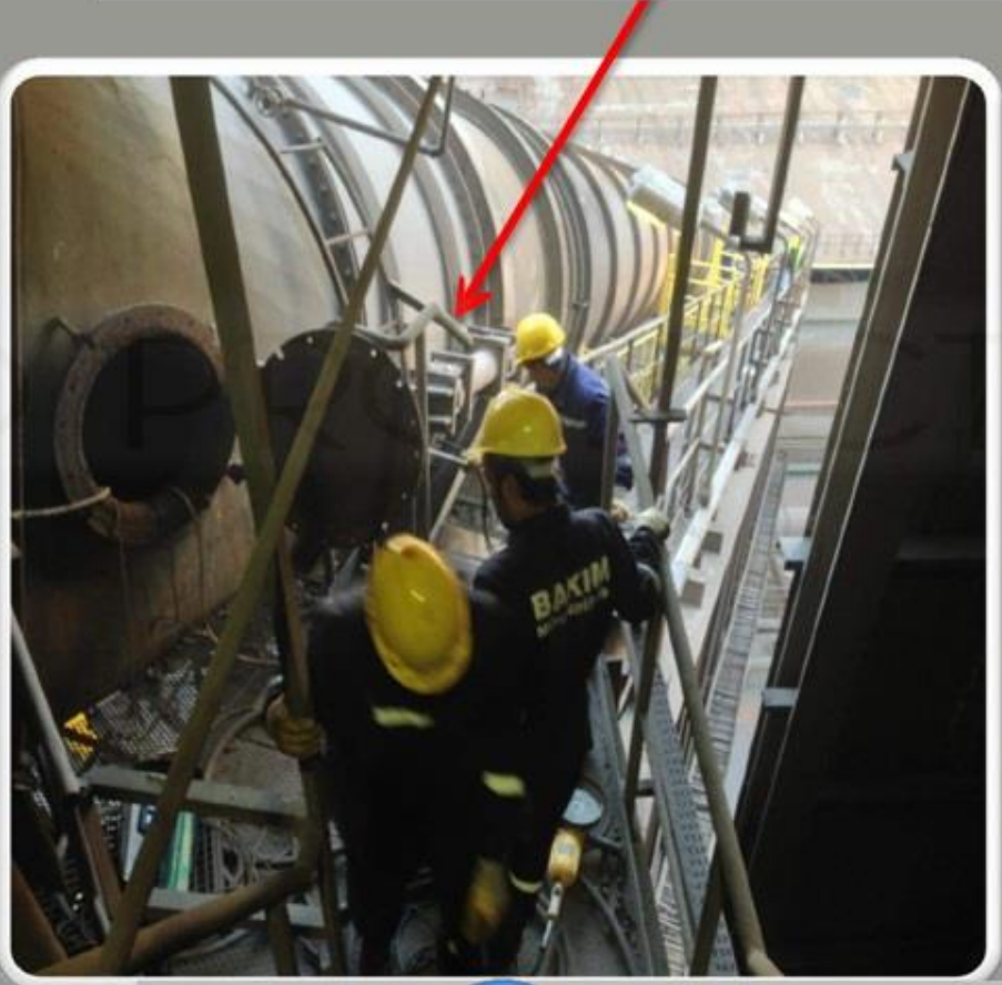
İsdemir Yatay Baca Konvertör Gaz Yıkama Ünitesi
